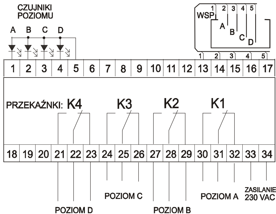
Rys. 03. Widok oraz listwa przyłączeniowa układu SPW-4-20 w obudowie IP20
