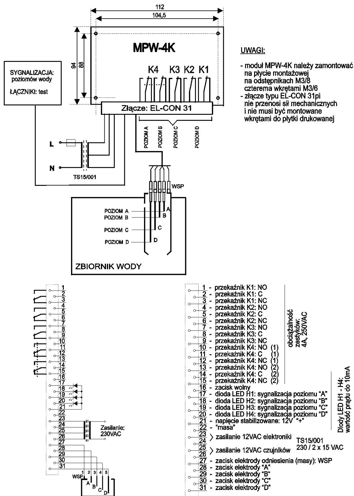
Rys. 01. Opis sygnałów na złączu płytki MPW-4K (przystosowanej do sygnalizatora 4-punktowego) - układ SPW-4-00
