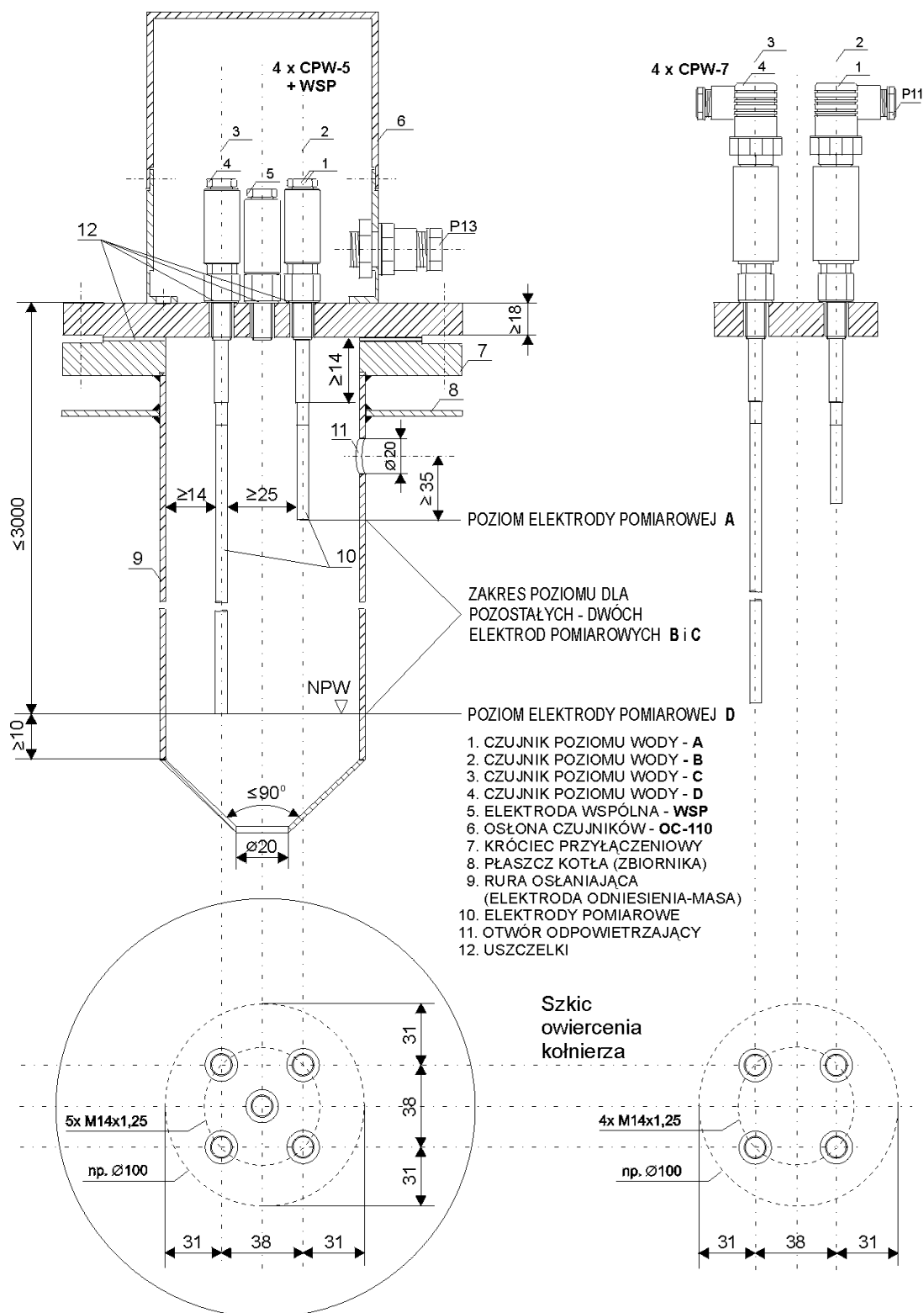
Rys.03. Sposób montażu konduktometrycznych czujników elektrodowych typ CPW-7 na króćcu przyłączeniowym zbiornika.
