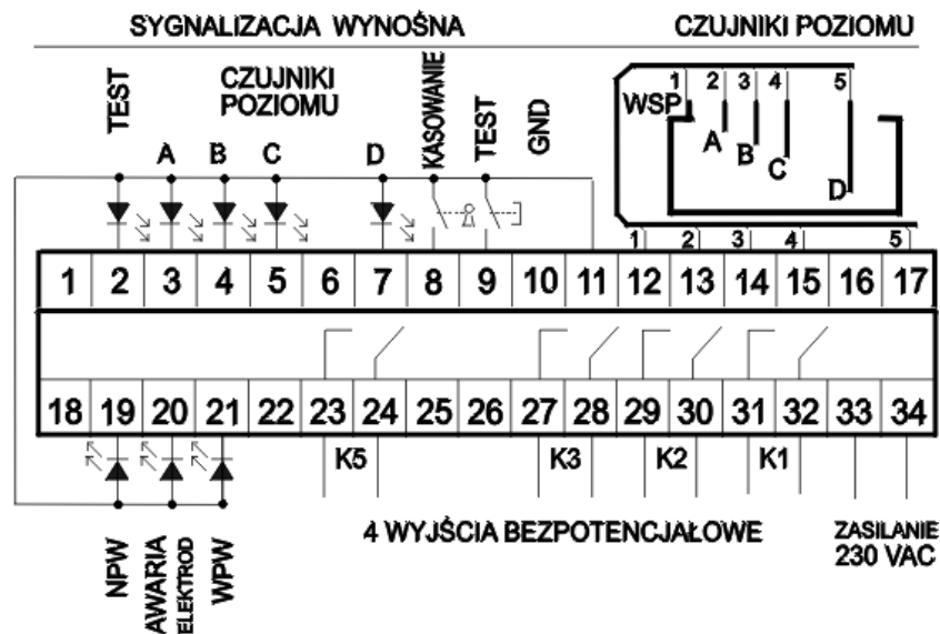
Rys.02. Widok oraz listwa przyłączeniowa układu MRPW-4v3-20 w obudowie IP20
