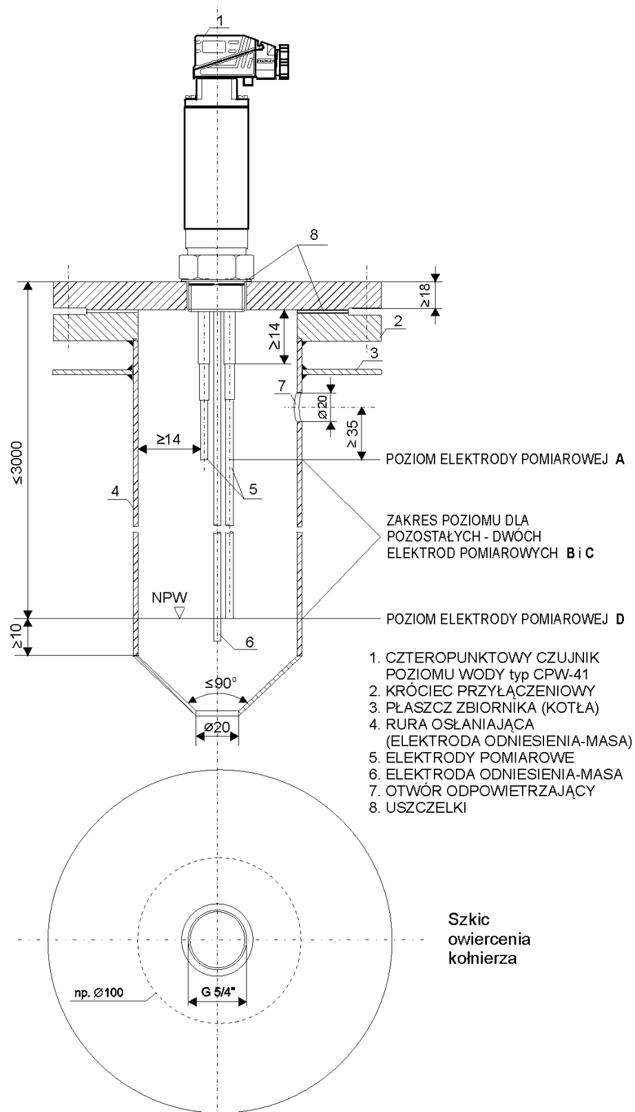
Rys.04. Sposób montażu czujnika 4-elektrodowego CPW-41 na króćcu przyłączeniowym zbiornika.
