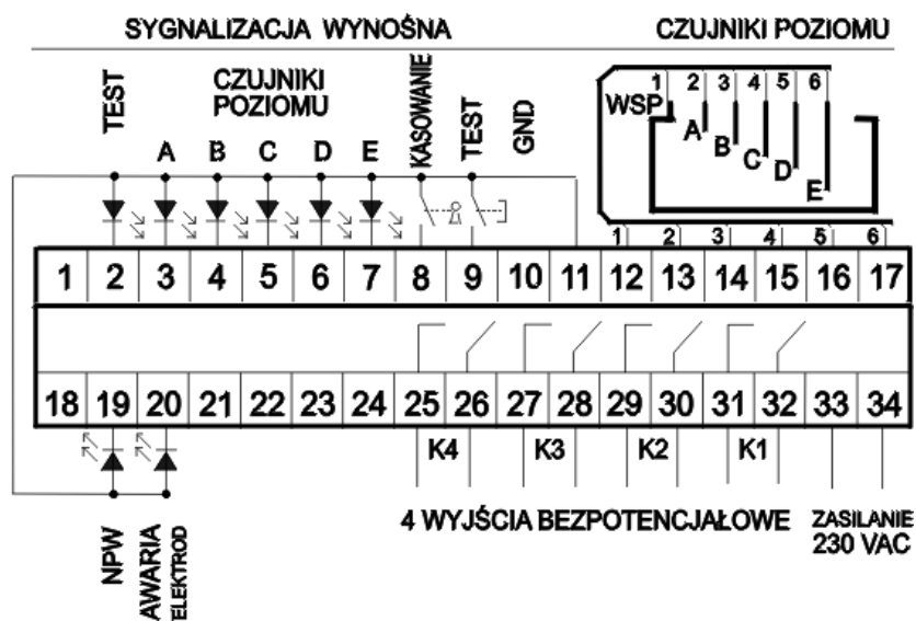
Rys.02. Widok oraz listwa przyłączeniowa układu MRPW-5v9-20 w obudowie IP20
