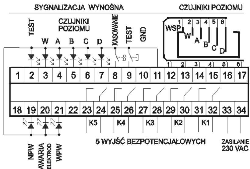
Rys.02. Widok oraz listwa przyłączeniowa układu MRPW-5v8-20 w obudowie IP20
