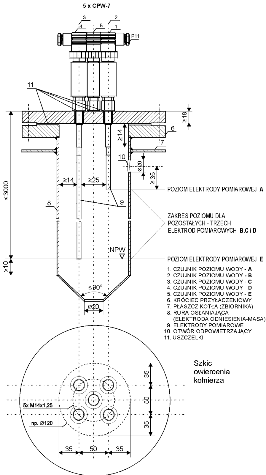
Rys.03. Sposób montażu konduktometrycznych czujników elektrodowych typ CPW-7 na króćcu przyłączeniowym zbiornika.
