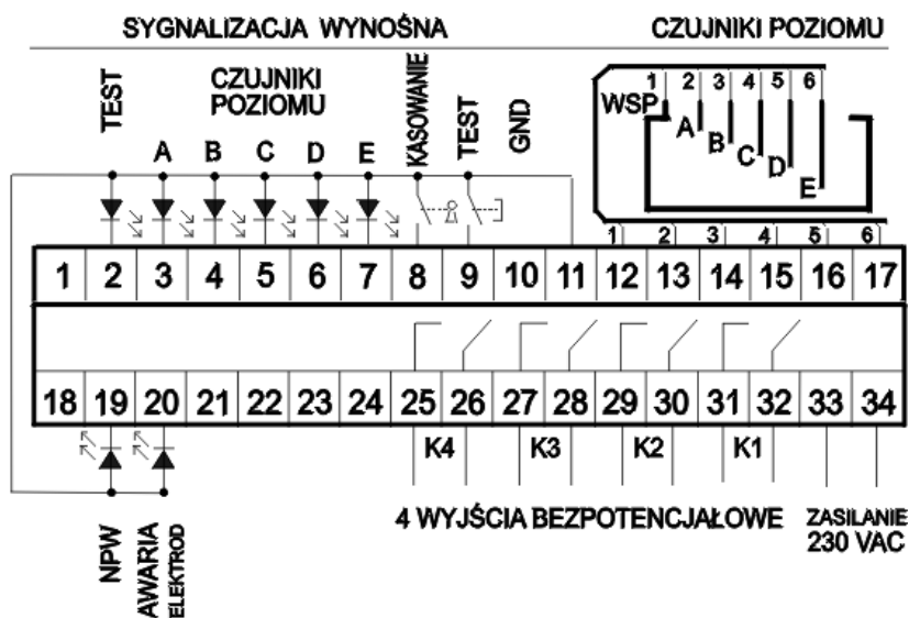
Rys.02. Widok oraz listwa przyłączeniowa układu MRPW-5v7-20 w obudowie IP20
