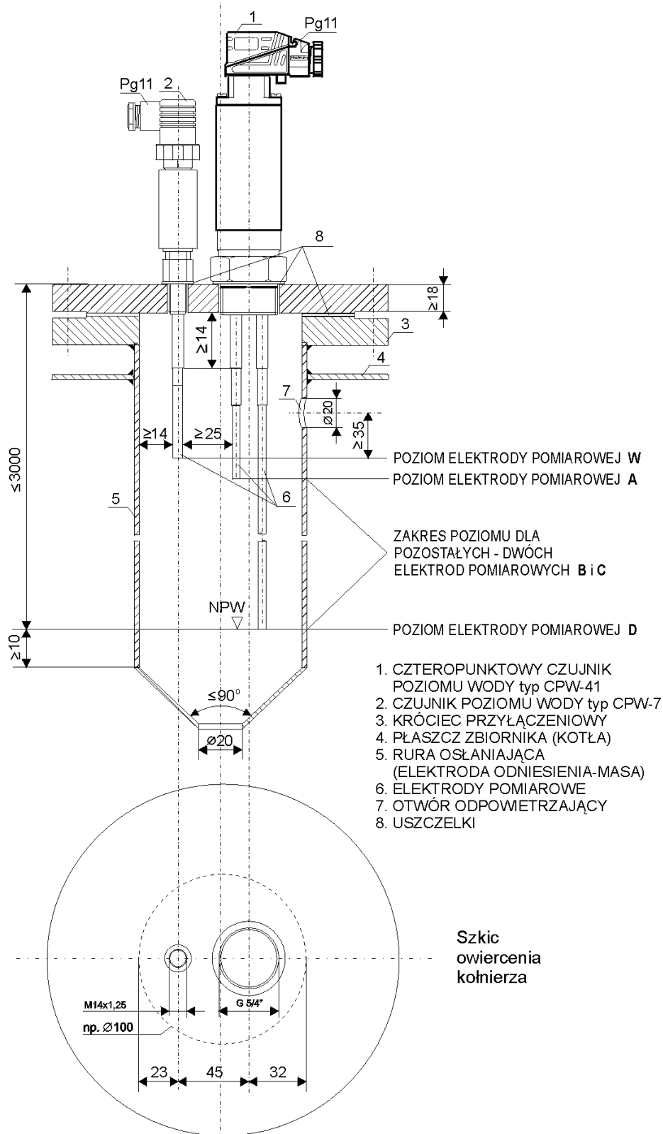
Rys.04. Sposób montażu zestawu konduktometrycznego czujnika elektrodowego CPW-7 oraz czujnika 4-elektrodowego CPW-41 na krótcu przyłączeniowym zbiornika.
