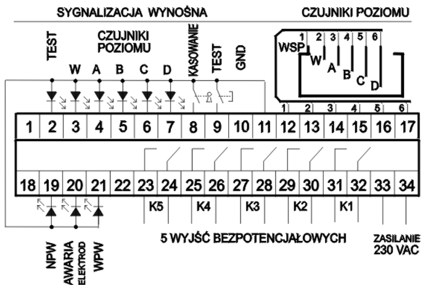
Rys.02. Widok oraz listwa przyłączeniowa układu MRPW-5v4-20 w obudowie IP20.
