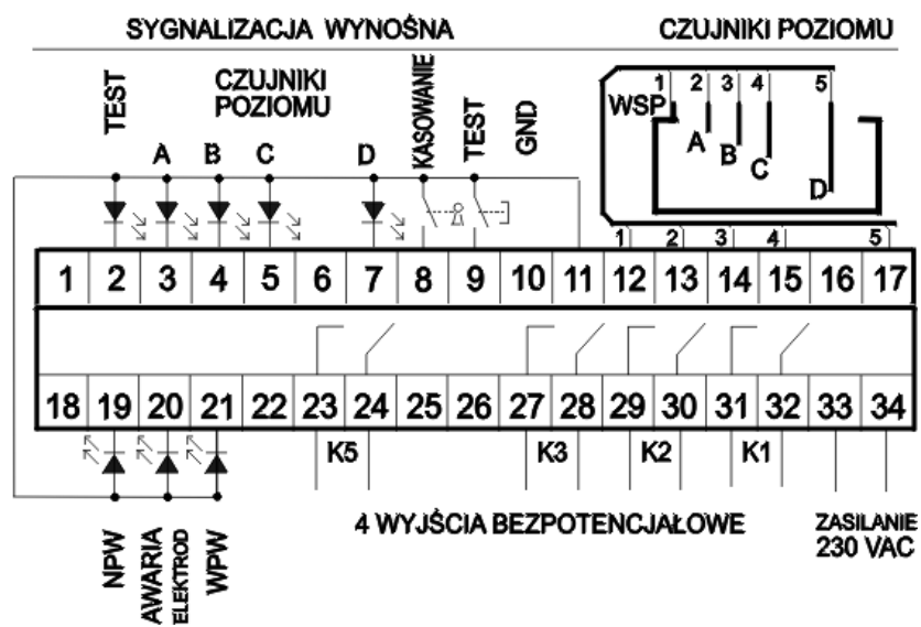
Rys.02. Widok oraz listwa przyłączeniowa układu MRPW-4V4-20 w obudowie IP20
